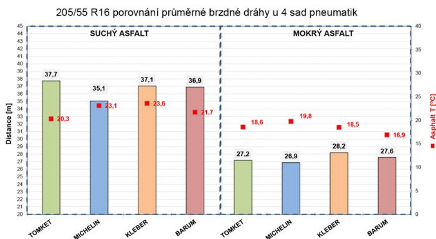
Graph 1: Brzdná dráha
