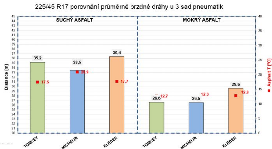
Graph 2: Brzdná dráha
