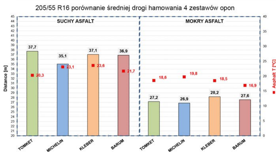
Graph 1: Droga hamowania
