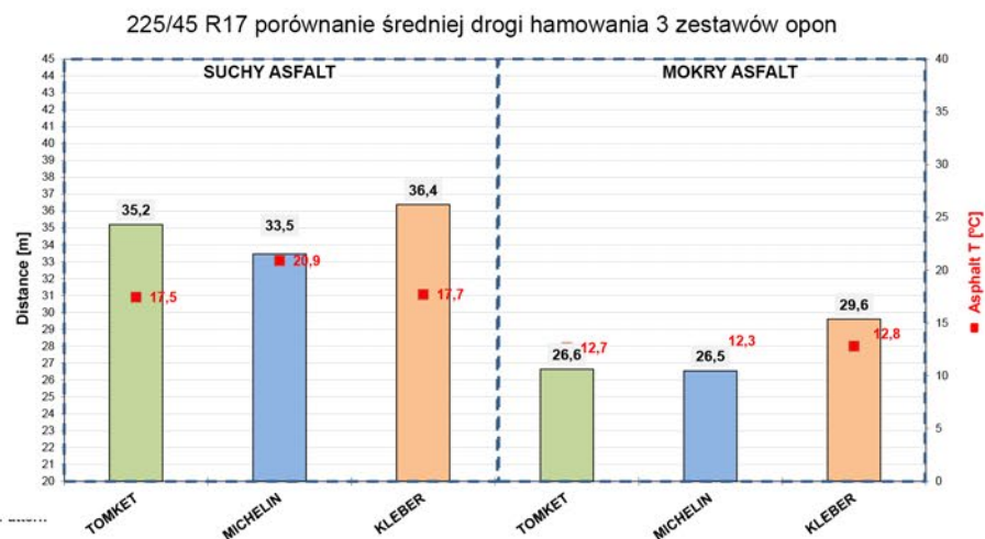
Graph 2: Droga hamowania
